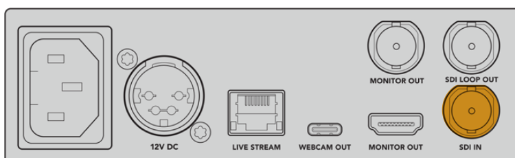
Podłącz wideo do wejścia SDI w Blackmagic Web Presenter
