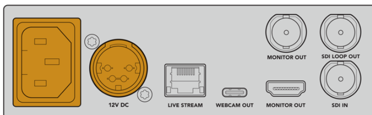
El dispositivo puede alimentarse mediante el cable IEC o una fuente de 12 V para corriente continua.
