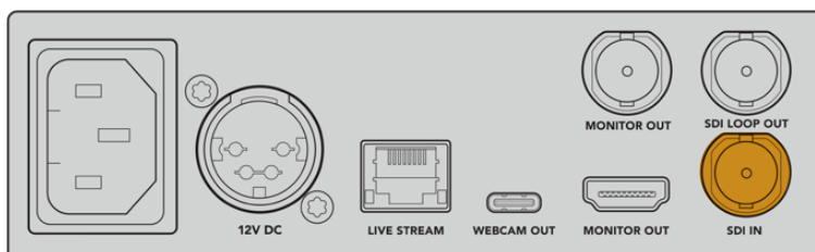
Connectez la vidéo à l'entrée SDI du Blackmagic Web Presenter.
